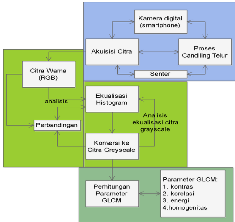
Gambar 4. Alur Proses Analisis GLCM pada Fertilitas Telur
