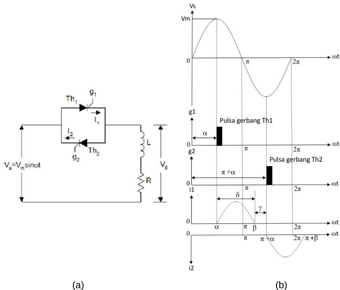
Gambar 1. Pengendali Tegangan 1-Fase dengan Thyristor : (a) Rangkaian, (a) Bentuk Gelombang Tegangan Sumber, Pulsa Pemicu, dan Arus yang Lewat Thyristor
