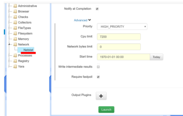
Fig. 11. Launching ArtifactCollectorFlow: Netstat
