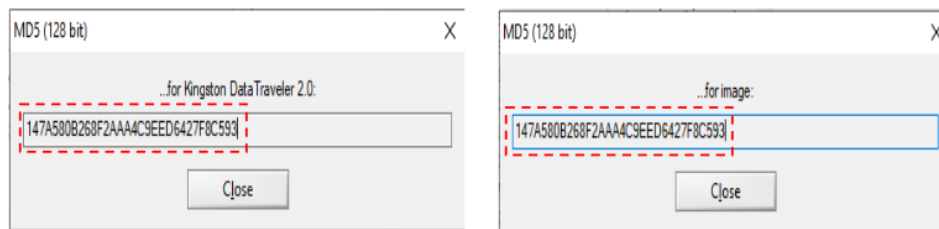
Gambar 7. Pencocokan nilai hash
