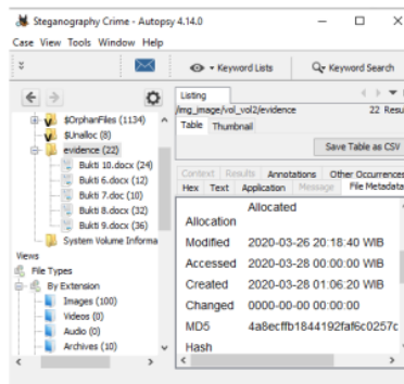
Gambar 10. Informasi metadata folder “evidence”
