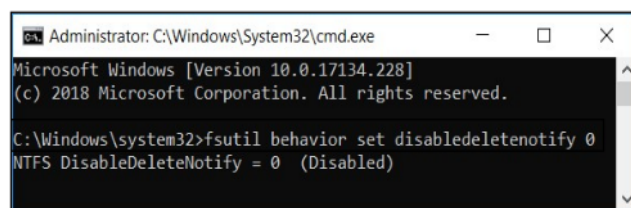
Gambar 7. Perintah TRIM enable di CMD
