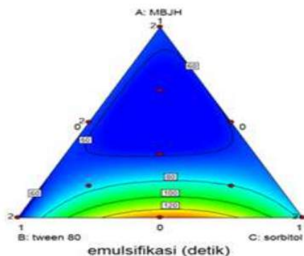
Gambar 2. Contour Plot Waktu Emulsifikasi
