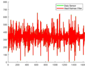
Gambar 3. R=1 Q=100
