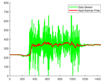
Gambar 11. Pengujian 3
