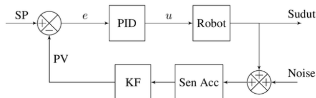
Gambar 2. Diagram Blok Kendali Sistem Kendali Kalang Tertutup
