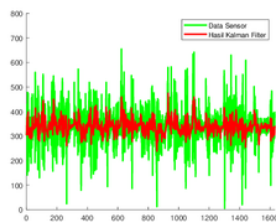
Gambar 6. R=1 Q=0,1
