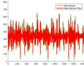
Gambar 4. R=1 Q=10
