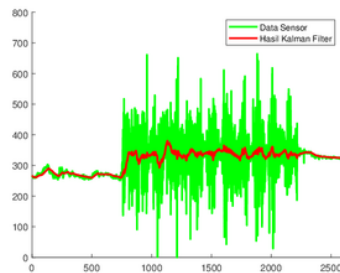
Gambar 9. Pengujian 1
