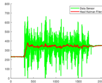
Gambar 10. Pengujian 2
