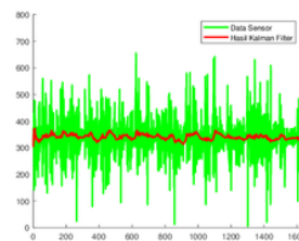
Gambar 8. R=10 Q=0,01
