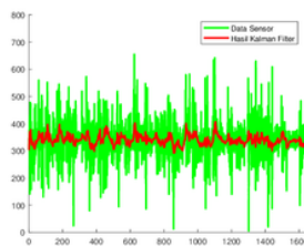
Gambar 7. R=10 Q=0,1
