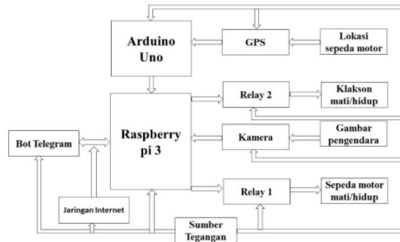
Gambar 2. Diagram Blok Perancangan Sistem
