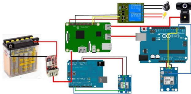
Gambar 3. Diagram Pengkabelan Sistem
