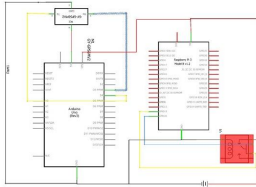
2 Gambar 4. Diagram Pengkabelan Sistem Dengan IC
