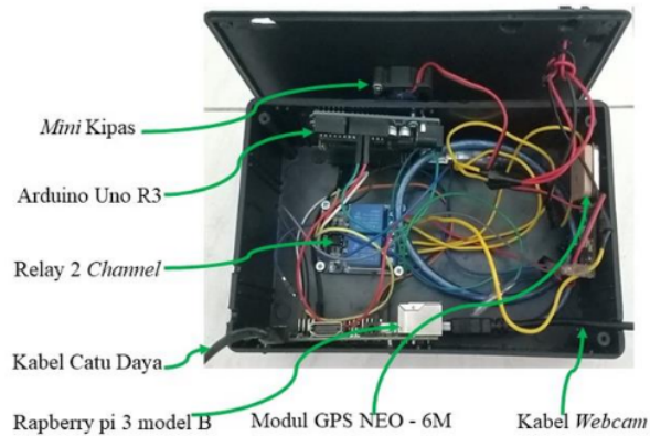
Gambar 7. Hardware sistem beserta letak komponennya
