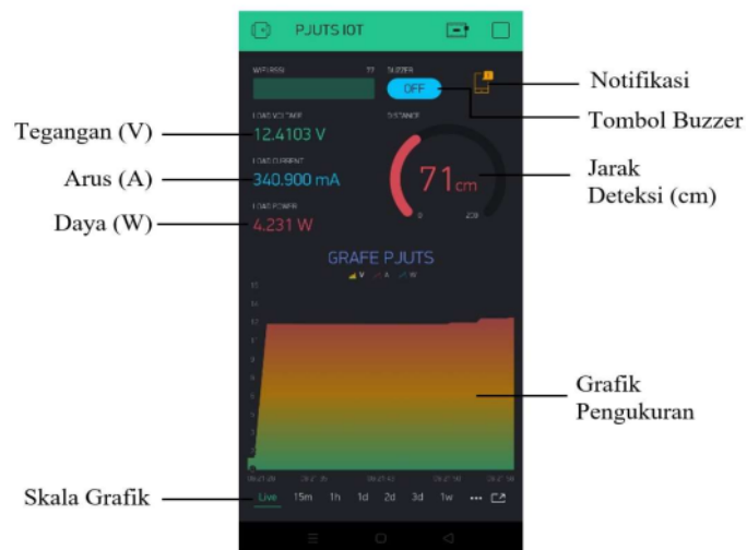
Gambar 9. Interface Aplikasi Blynk
