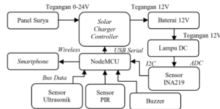
Gambar 2. Diagram Blok Perancangan Sistem
