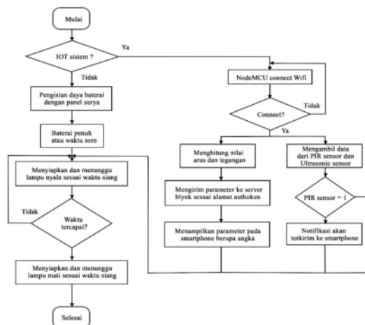
Gambar 6. Diagram Alir Proses Pembacaan dan Pengiriman data
