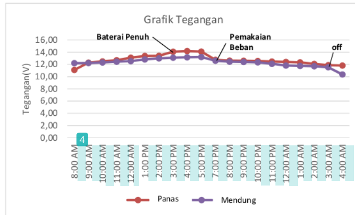
Gambar 7. Grafik voltase terhadap waktu
