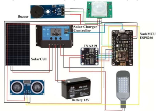
Gambar 3. Diagram Perancangan Sistem
