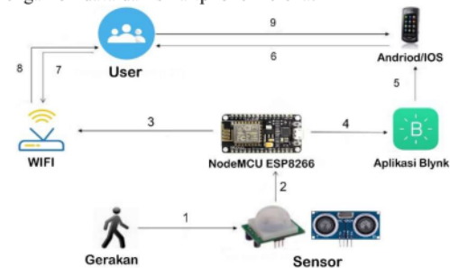
Gambar 11. Sistem pendeteksi pergerakan
