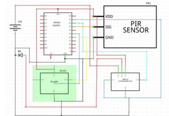
Gambar 4. Diagram Rangkaian Pengkabelan Sistem
