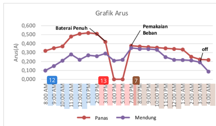
Gambar 8. Grafik arus terhadap waktu
