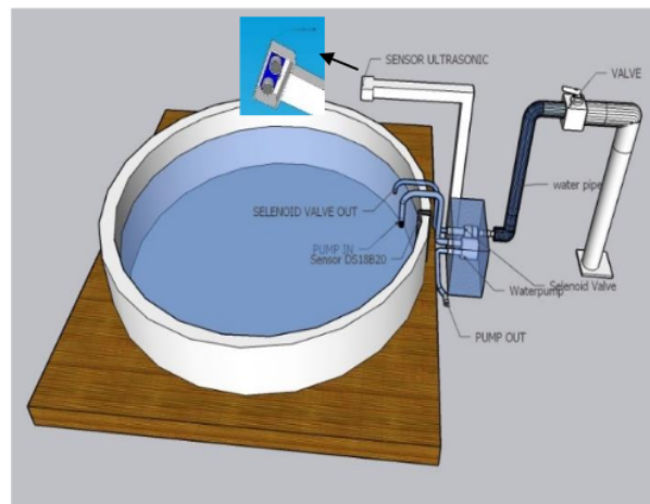
Gambar 6. Desain Alat
