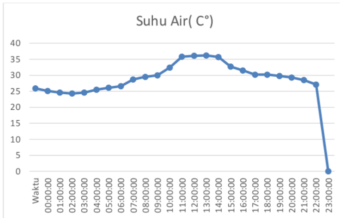
Gambar 9. Grafik data suhu air
