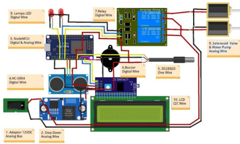
Gambar 4. Diagram pengkabelan alat
