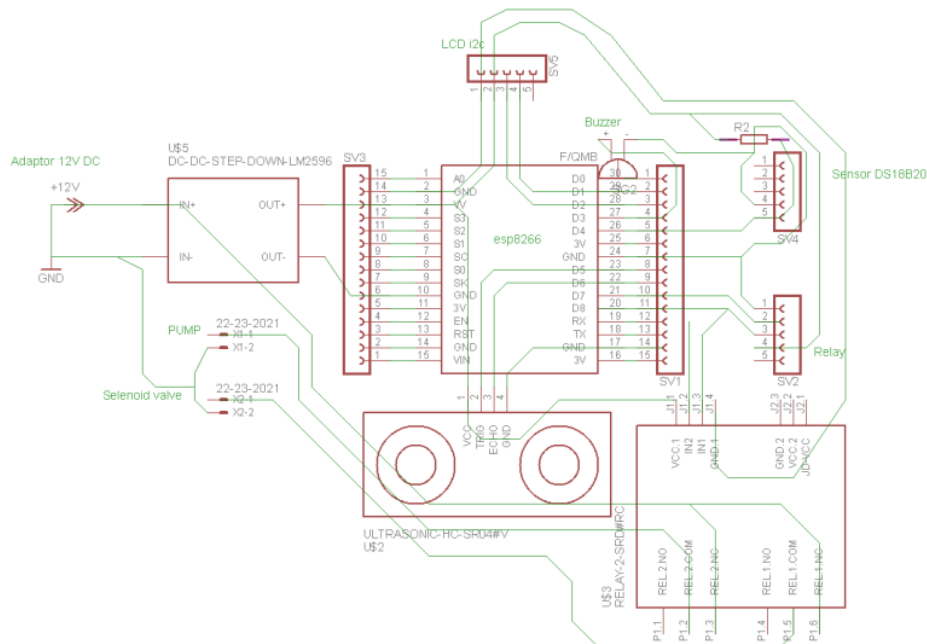
Gambar 3. Rangkaian keseluruhan alat
