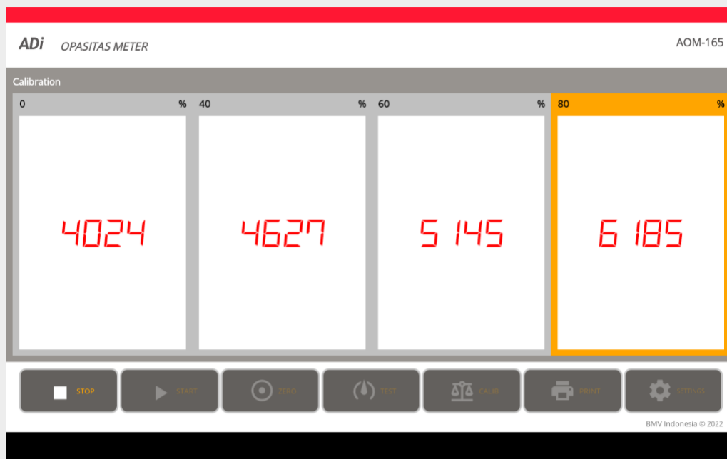
Tampilan kalibrasi 80
