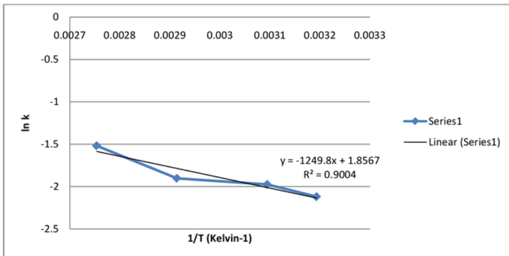
Gambar 2 Grafik hubungan 1/T dengan ln k
