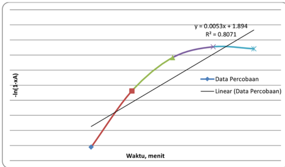
Gambar 1. Grafik hubungan waktu dan -\ln(1-X_a)
