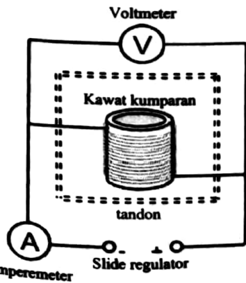
Gambar 2. Skema rangkaian alat eksperimen
