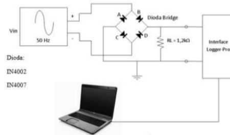
Gambar 1. Skema eksperimen penentuan kualitas rangkaian penyearah gelombang penuh
