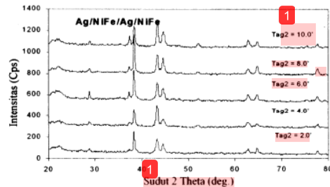
Gambar 2. Intensitas Ag, NiO, NiFe dan Fe_2O_3 terhadap sudut difraksi 2 theta
