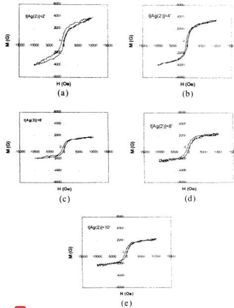
1 Gambar 4. Kurva loop histeresis sistem multilapisan Ag/NiFe/Ag/NiFe pada berbagai t_{Ag(2)} : (a) untuk t_{Ag(2)} = 2 menit, (b) untuk t_{Ag(2)} = 4 menit, (c) untuk t_{Ag(2)} = 6 menit, (d) untuk t_{Ag(2)} = 8 menit, (e) untuk t_{Ag(2)} = 10 menit
