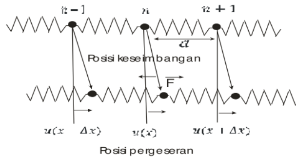
Gambar 1 Kisi-kisi monoatomik pada posisi keseimbangan dan pergeseran
