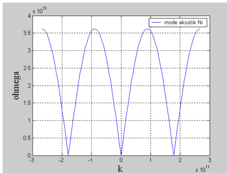
Gambar 3 Kaitan Dispersi Atom Ni dengan beberapa nilai k
