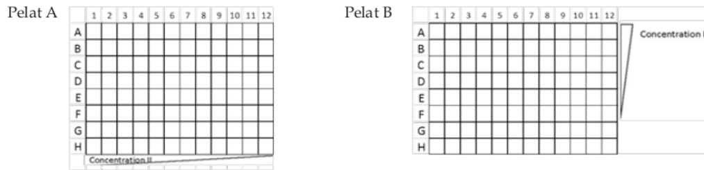
Gambar 1 Pola pengisian sampel dalam sumuran serta konsentrasinya
