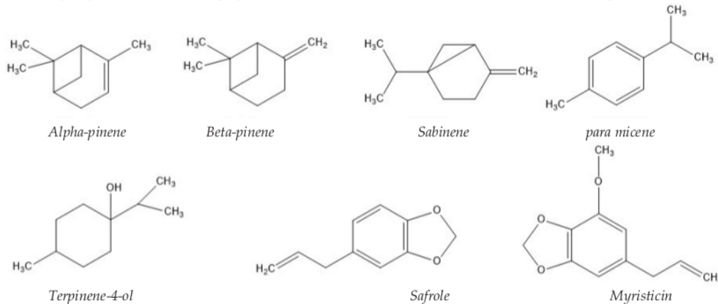
Gambar 5 Struktur komponen utama minyak atsiri (A) Syz; dan (B) Myr
