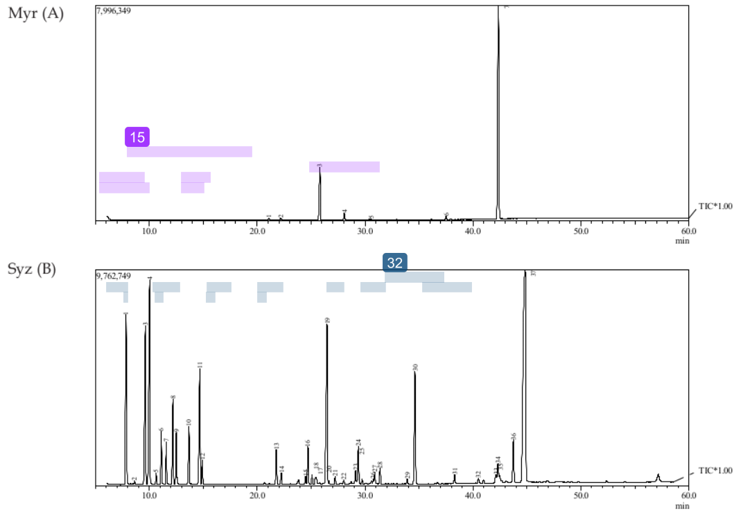
Gambar 4 Profil kromatogram GC-MS minyak atsiri kedua senyawa uji (A) Myr dan (B) Syz
