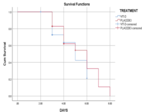
Gambar 1. Kurva Kaplan Meier
