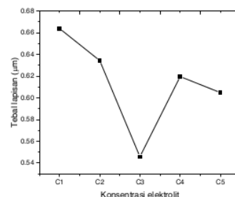
Gambar 1. Grafik hubungan tebal lapisan dan konsentrasi elektrolit
