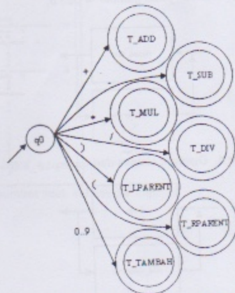
Gambar 3. Rancangan scanner dengan Finite Automata
