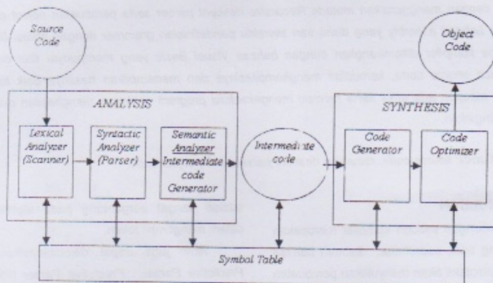
Gambar 1. Model kompilier
