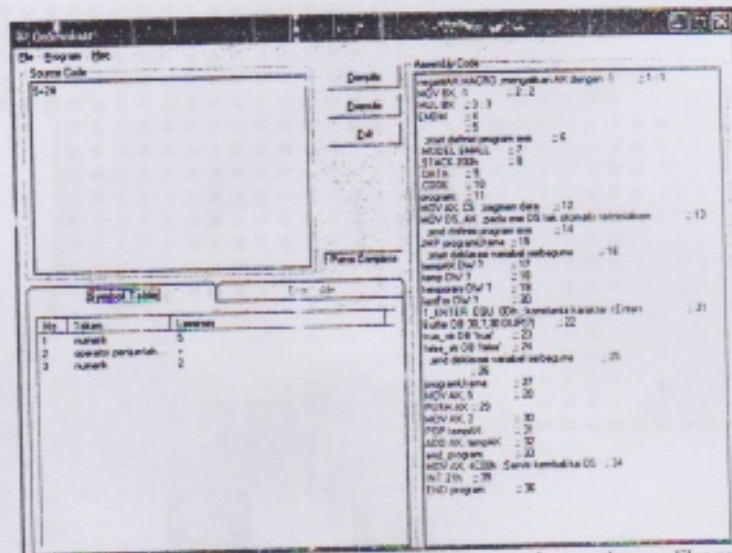
Gambar 6. Tampilan program sewaktu kode sumber sukses dikompilasi
