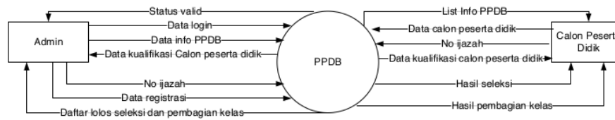
Gambar 1. DFD level 0 Sistem Penerimaan Peserta Didik Baru
