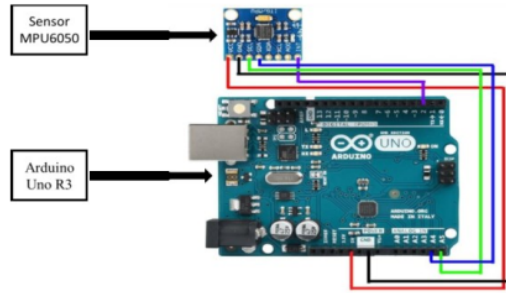
Fig. 2. Wiring diagram
