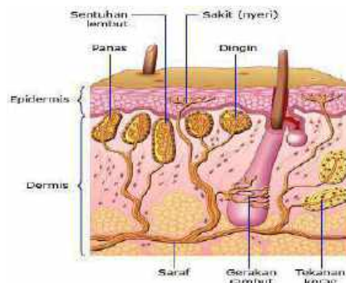
Gambar 12. Anatomi kulit
