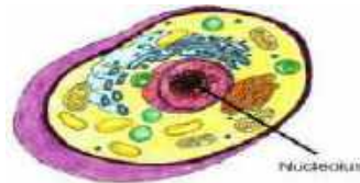
Gambar 14. Nukleolus
