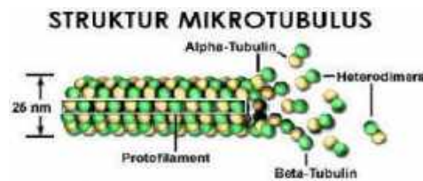
Gambar 12. Mikrotubulus
