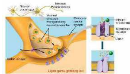
Gambar 3. Sinapsis
