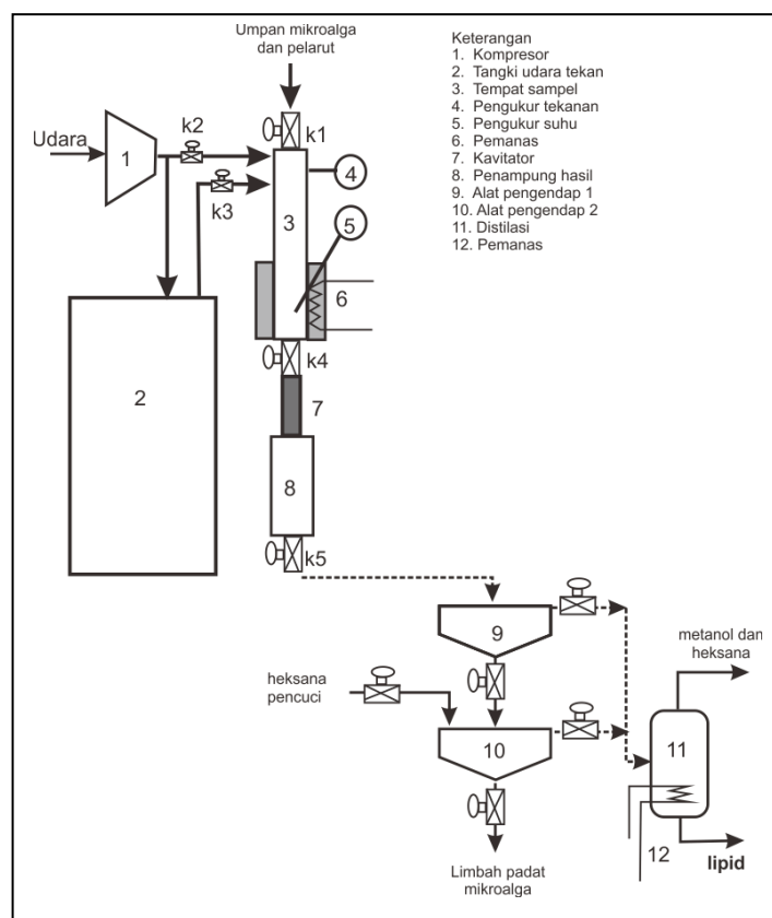
Gambar 1. Skema alat penelitian ekstraksi kavitasi hidrodinamika
