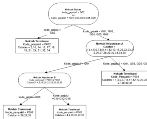
Gambar 6 Pohon Keputusan Iterasi 3
