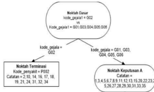
Gambar 4. Pohon Keputusan Iterasi 1
