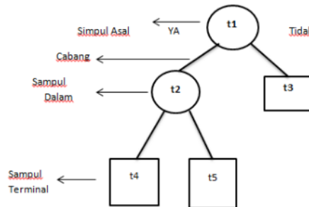
Gambar 2 Skema Cabang Pohon CART [19]
