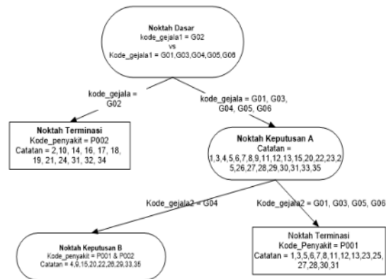
Gambar 5 Pohon Keputusan Iterasi 2
