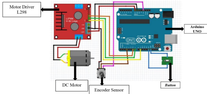
Fig. 3. Wiring Hardware
