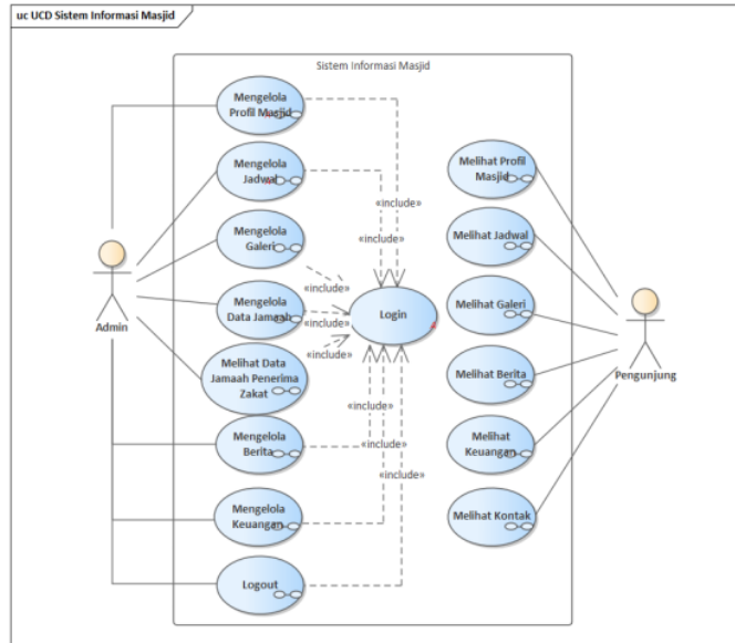
Gambar 3. Use Case Diagram Sistem Informasi Masjid
