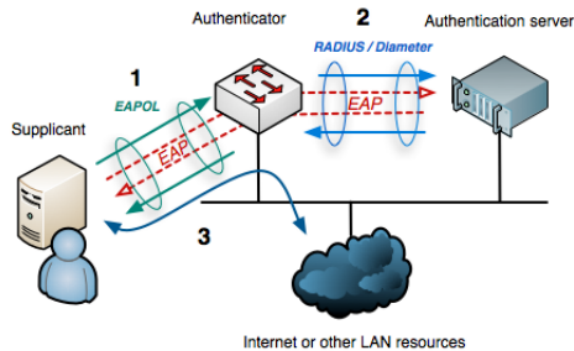
Gambar 1. Topologi protokol 801.2X
