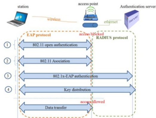
Gambar 2. Ilustrasi otentikasi 802.1X
