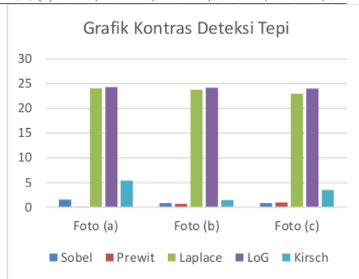
Gambar 9. Grafik Nilai Kontras Deteksi Tepi
