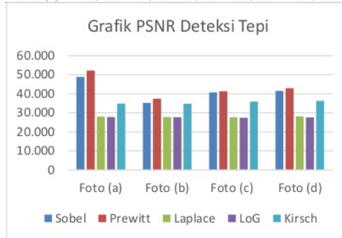
Gambar 7. Grafik Nilai PSNR Deteksi Tepi
