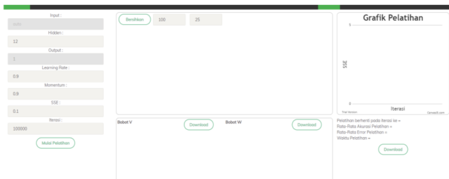
Gambar 6. Antarmuka halaman pelatihan sistem prediksi
