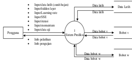
Gambar 5. Diagram Alir Data Sistem Prediksi
