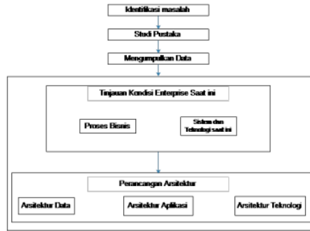
Gambar 3. Kerangka Penelitian
