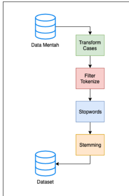
Gambar 1. Tahap Pemrosesan Teks
