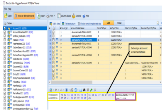
Gambar 4 akun email Google Drive yang di hapus
