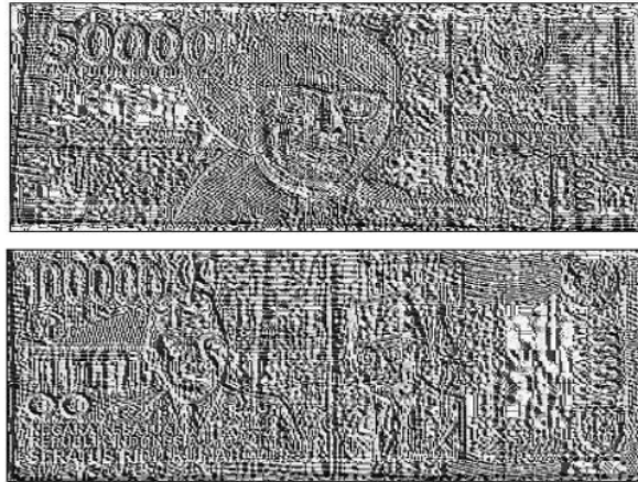
Gambar 4. Tekstur LBP
