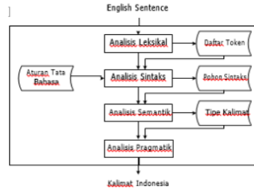
Gambar 2.1 komponen bahasa alami (Raharjo & Hartati, 2014)
