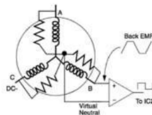
Gambar 2. Rangkaian komparator sederhana dengan menerapkan titik virtual neutral [2].
