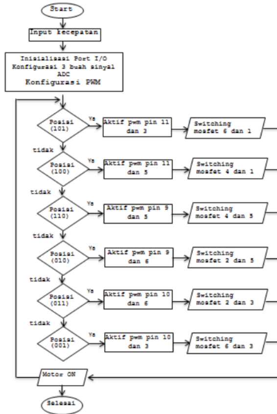
Gambar 4. Diagram alir kendali motor BLDC tanpa sensor
