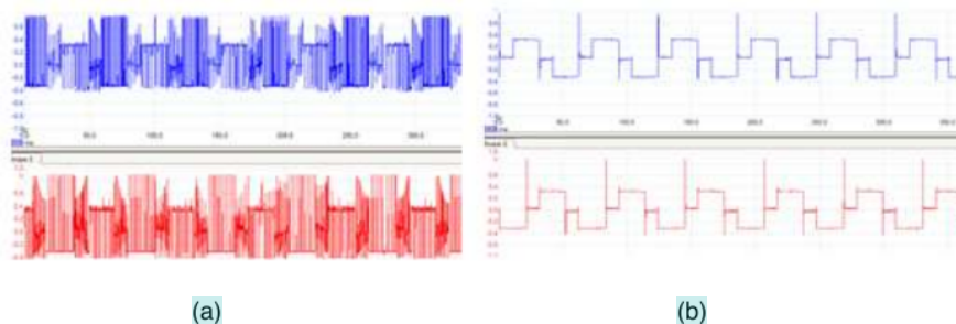
Gambar 14. Sinyal inverter dengan beban yang dikeluarkan pada terminal daya, (a) Output sinyal inverter dengan PWM 150 (b) Output sinyal inverter dengan PWM 255
