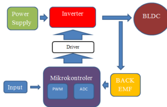
Gambar 1. Diagram sistem kontrol BLDC tanpa sensor
