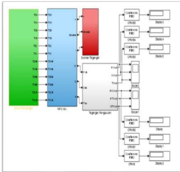
Gambar 2. Rangkaian NPC-MLI secara keseluruhan
