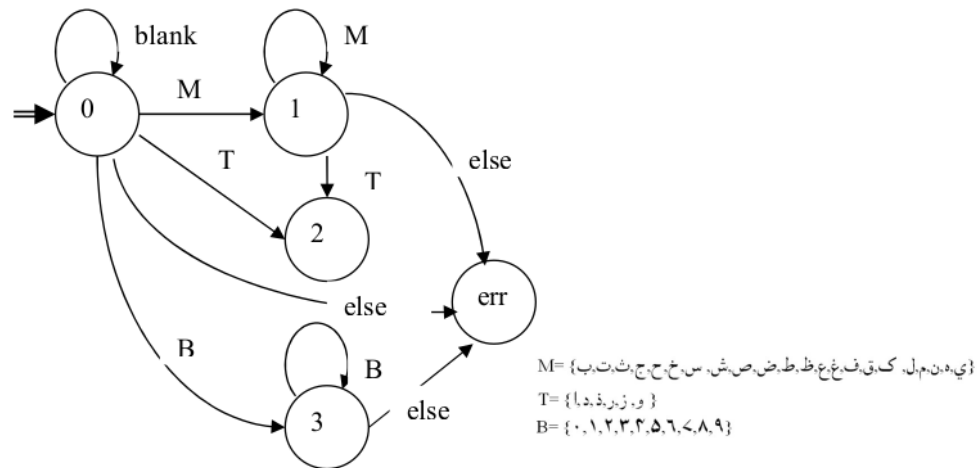
Gambar 8. FSA susunan huruf Hijaiyyah
