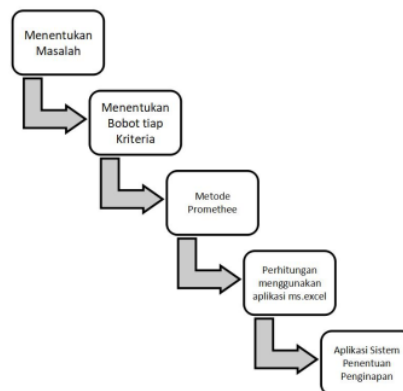
Gambar 1. Tahapan Penelitian
