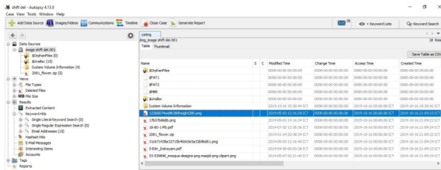
Gambar 9. Hasil Examination menggunakan Autopsy pada SD Card dengan cara hapus Shift+Delete.
