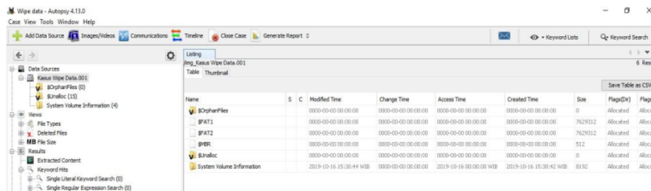
Gambar 10. Hasil Examination menggunakan Autopsy pada SD Card dengan cara hapus Wipe Data.
