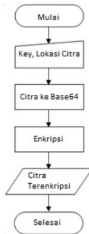
Gambar 3 Diagram Alir Proses Enkripsi
