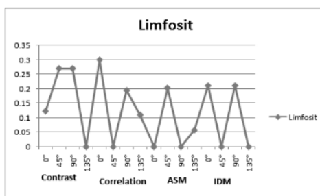
Gambar 14. Hasil Klasifikasi Sel Limfosit
