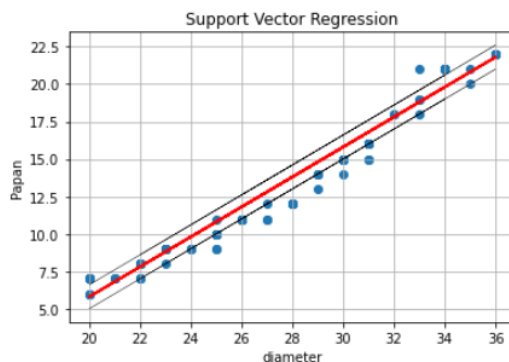
Gambar 3: Hasil SVR
