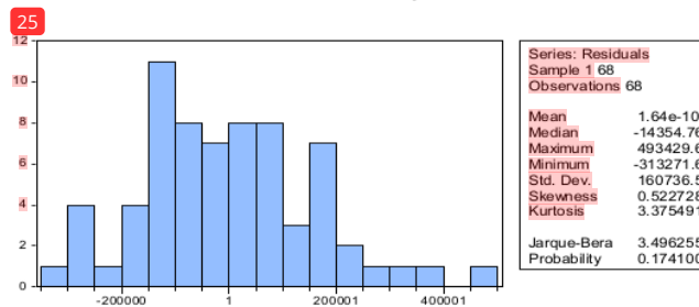
Gambar 1. Pengujian Normalitas
