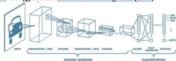
Gambar 2. Proses pada CNN
