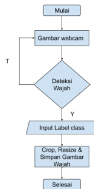
Gambar 7. Alur pengambilan dataset wajah
