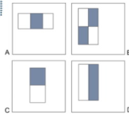
Gambar 1. Fitur Haar
