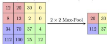
Gambar 4. Layer maximum pooling
