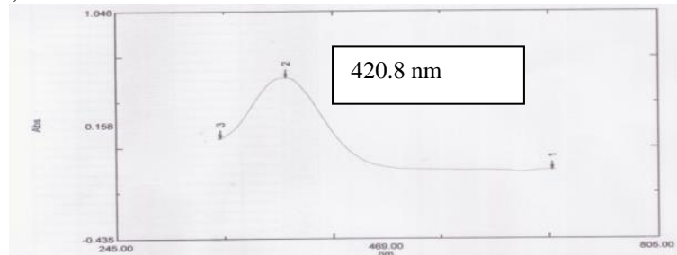
Gambar 2. Panjang gelombang pada absorbansi maksimum kompleks reserpin BCG konsentrasi 25 µg/ml
