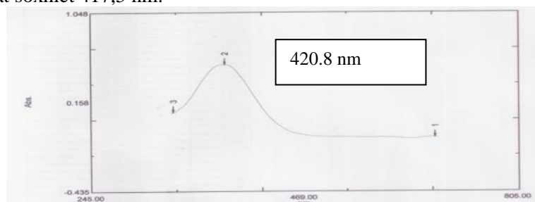
Gambar 2. Panjang Gelombang Pada Absorbansi Maksimum Kompleks Reserpine BCG Konsentrasi 25 µg/ml
