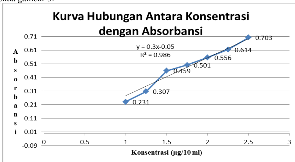
Gambar 3. Kurva Hubungan Antara Konsentrasi Reserpin ( \mu\text{g}/10\text{ml} ) dengan Absorbansi
