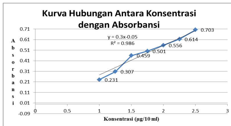
Gambar 3. Kurva hubungan antara konsentrasi reserpin (µg/ 10mL) dengan absorbansi
