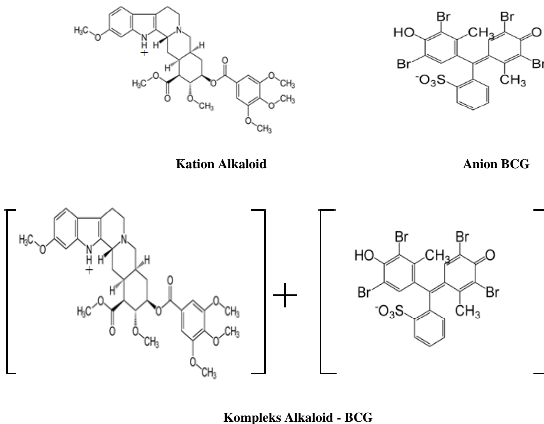
Gambar 1. Reaksi Pembentukan Kompleks Antara Reserpine dengan BCG
