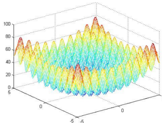
Fig. 1. Rastrigin function
