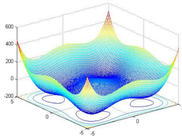
Fig. 5. 2^n minima function
