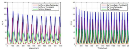
Gambar 5. Simulasi numerik b=2.5 dan b=3 .
