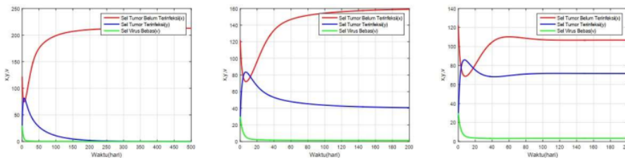
Gambar 2. Simulasi numerik b=0.1, b=0.2, \text{ dan } b=0.3.
