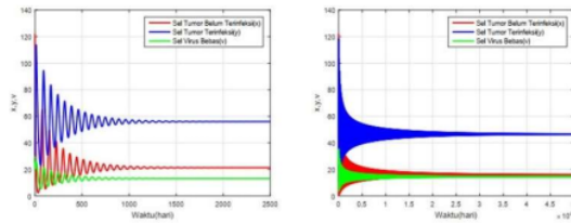
Gambar 4. Simulasi numerik b=1.5 dan b=2 .
