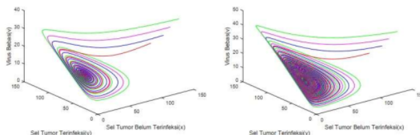
Gambar 8. Potret fase sistem untuk b=1.5 dan b=2 .
