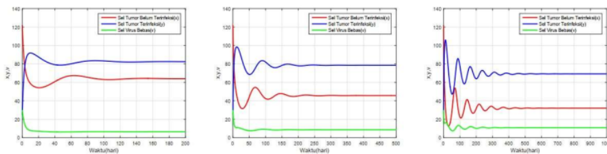
Gambar 3. Simulasi numerik b=0.5, b=0.7 \text{ dan } b=1.
