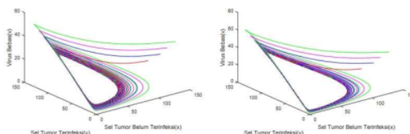
Gambar 9. Potret fase sistem untuk b=2.5 dan b=3 .
