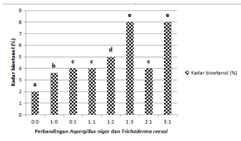
Gambar 2. Kadar bioetanol kulit mangga setelah fermentasi dengan menggunakan Saccharomyces cerevisiae angka pada gambar yang diikuti huruf yang sama menunjukkan tidak ada beda nyata ( Duncan < 0,05 ).
