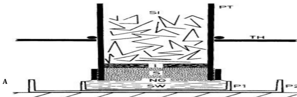
Gambar 3. Skema saringan Water ice treatment . I: Penyekat (Kapas), NG: Kasa Nilon ukuran 1000 \mu\text{m} , P1: Cawan petri (diameter 9 cm), P2: Cawan petri (diameter 15 cm), PT: Pipa paralon, S: Sedimen, SI: Pecahan es batu, SW: Air muara, TH: Statif (Uhlig et al. , 1973)
